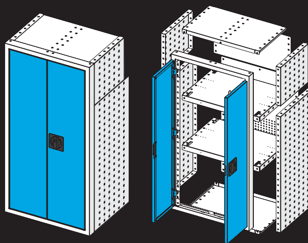
Stepped version for different depths Versión cortada a medida con escalón para cambio profundidad
