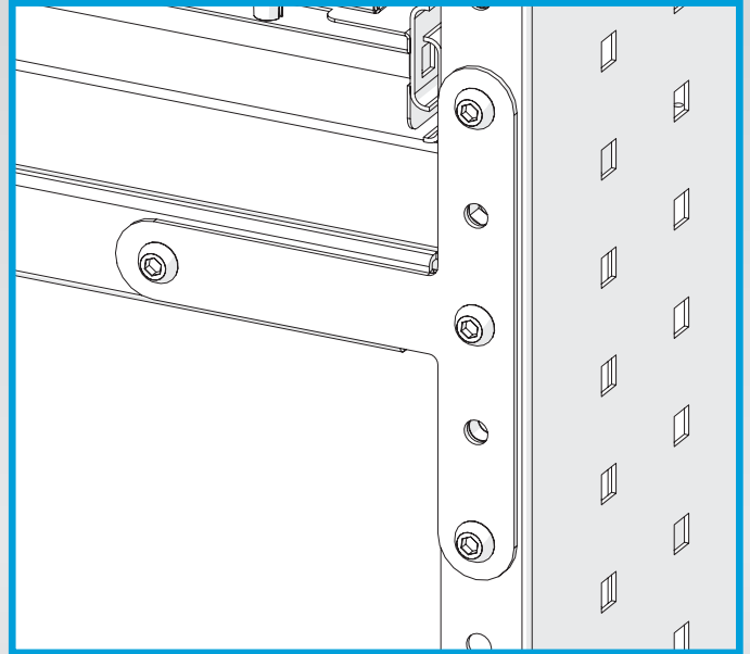
An ABC00004 bracket. Montaje refuerzo ABC00004.
