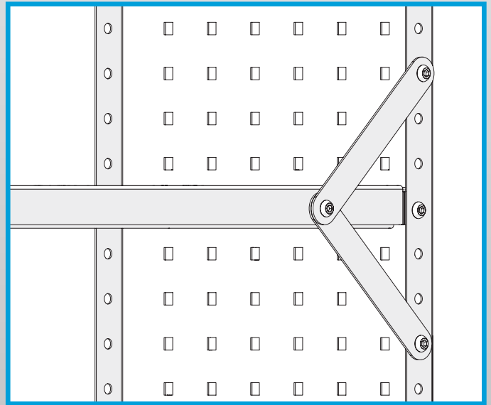
A pair of ABC00002 brackets facing up and down. Refuerzos ABC00002 montados en el mismo angular tanto hacia arriba como hacia abajo.
