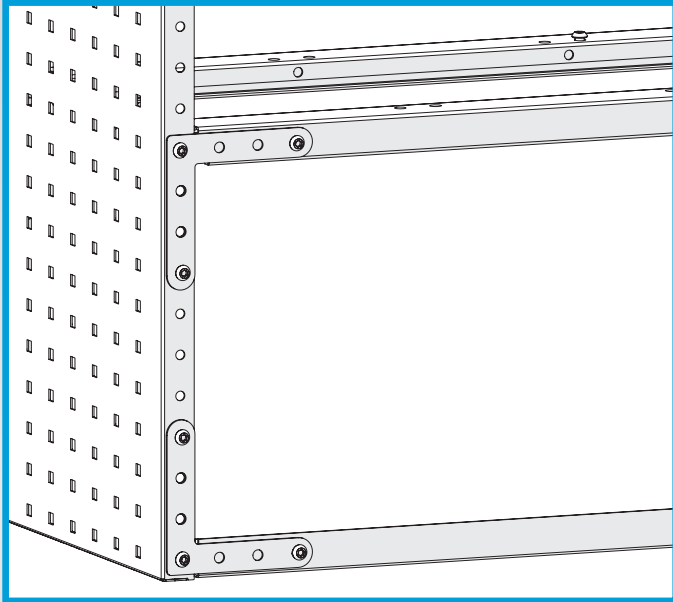
ABC00001 brackets facing up and down. Montaje refuerzos ABC00001 girados tanto hacia arriba como hacia abajo.
